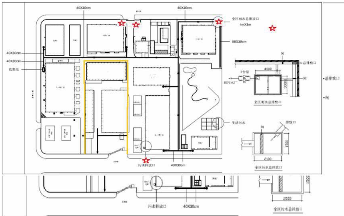
附件 6.4 雨水收集管网图
