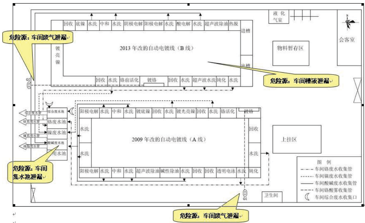
附件 6.1 平面布置及危险源分布图
