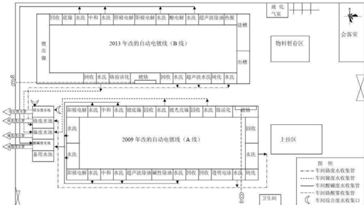
附件 6.3 污水收集管网图
